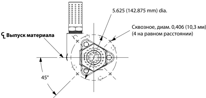
ВИД СНИЗУ
