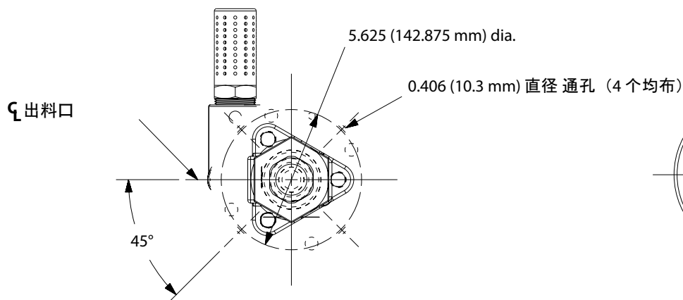
底视图
