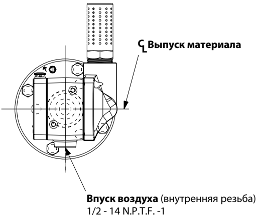
ВИД СВЕРХУ
