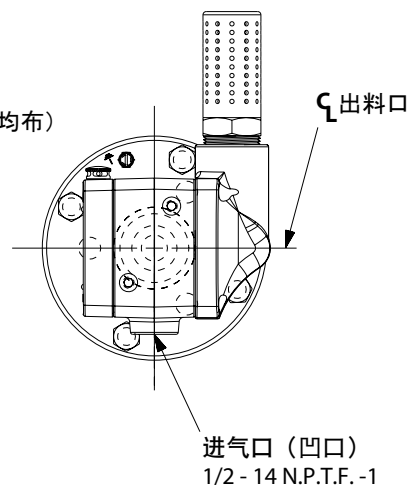
顶视图
