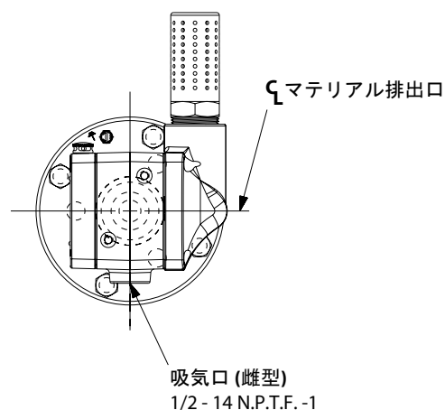
上部図
